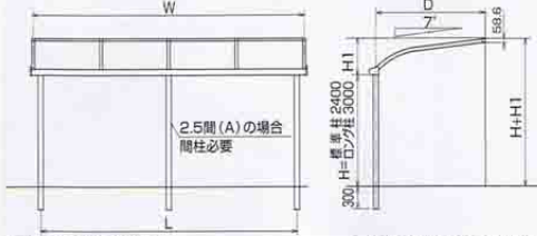
■基本タイプ寸法表
