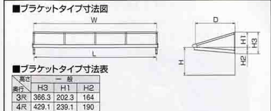
■ブラケットタイプ寸法表
