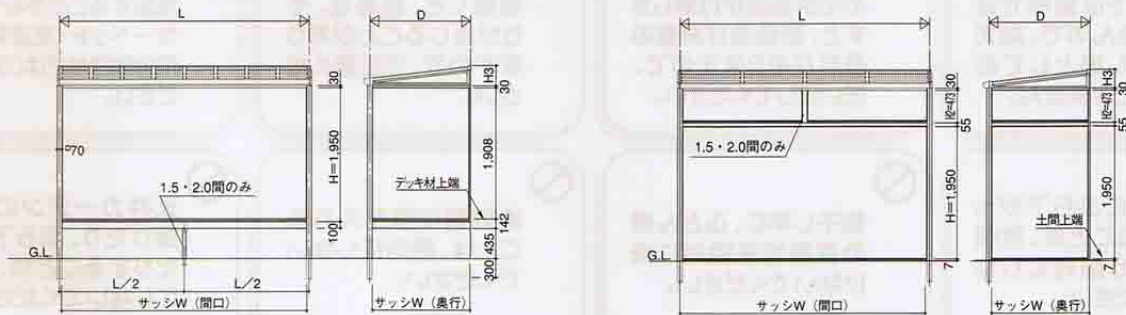
標準タイプ 積雪地域向 ランマ無 デッキ材仕様 | 土間タイプ 一般地域向 ランマ付
