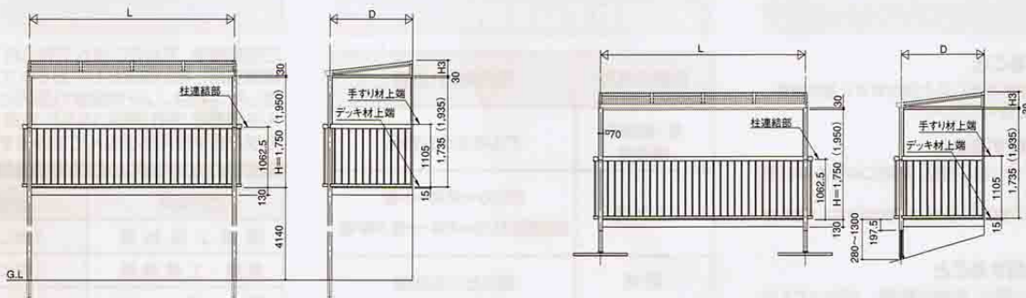
柱建タイプ 一般地域向 ランマ無 デッキ材仕様 | 屋根置タイプ 一般地域向 ランマ無 デッキ材仕様
