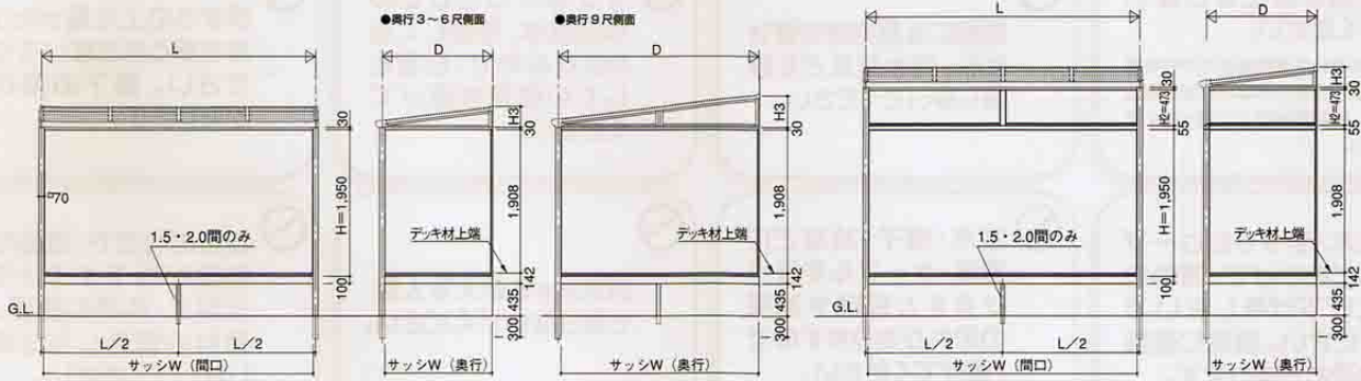
標準タイプ 一般地域向 ランマ無 デッキ材仕様 | ランマ付 デッキ材仕様
